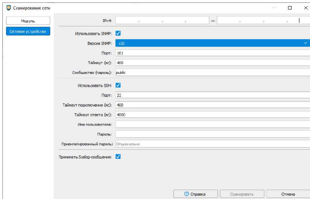
Рис. 284. Окно сканирование сети
